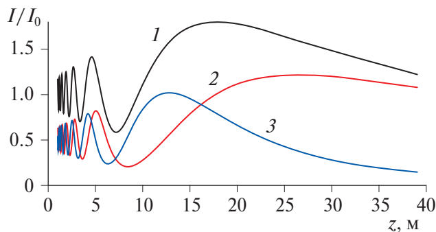
Рис. 2. Относительная интенсивность пучка СИ в центре щели в зависимости от расстояния до детектора ( I ) и вклады в нее от косинуса (2) и синуса (3) для d = 50 мкм и энергии фотонов 25 кэВ.
